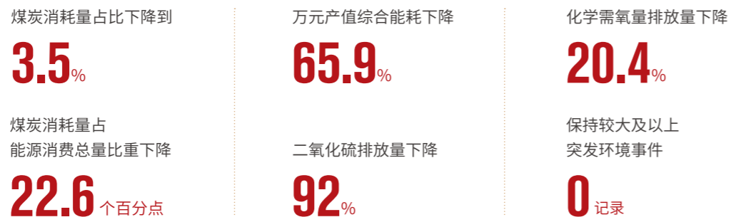
2013 — 2022 年环保数据对比
